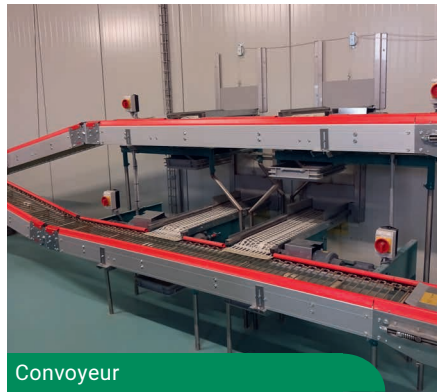
Convoyeur incliné
