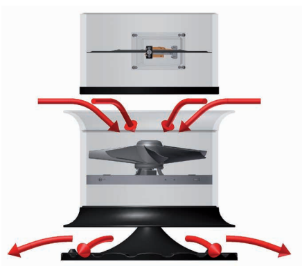
Niveau 1 Uniquement air de circulation Phase d'échauffement et de démarrage
