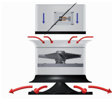
Niveau 2 Mélange d'air Phase de production
